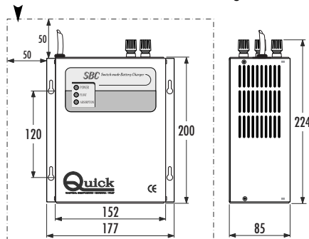
Abmessungen (mm)
