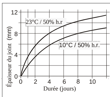
Diagramme 1 : Vitesse de polymérisation du Sikaflex®-291i
